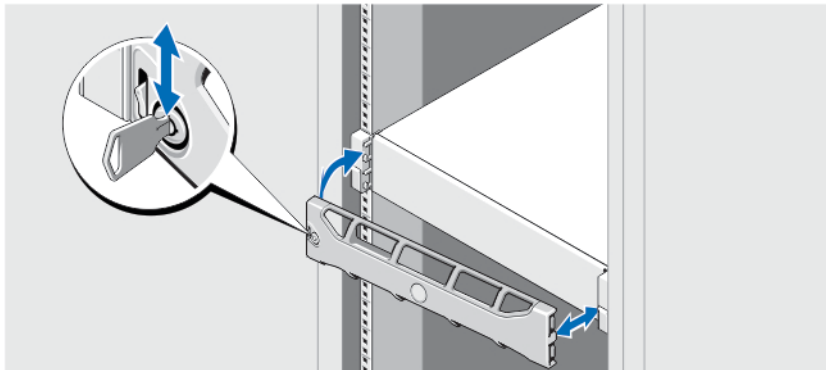
그림 6. 베젤 설치
