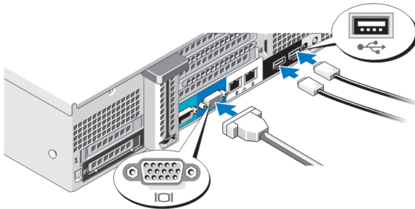
그림 2. 키보드, 마우스 및 모니터 연결
